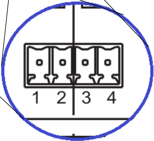
腳位配置
